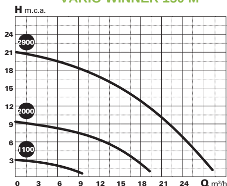
VARIO WINNER 150 M
