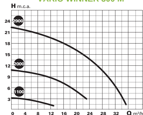
VARIO WINNER 300 M
