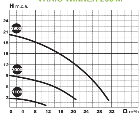
VARIO WINNER 200 M
