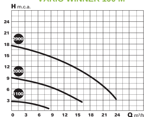
VARIO WINNER 100 M
